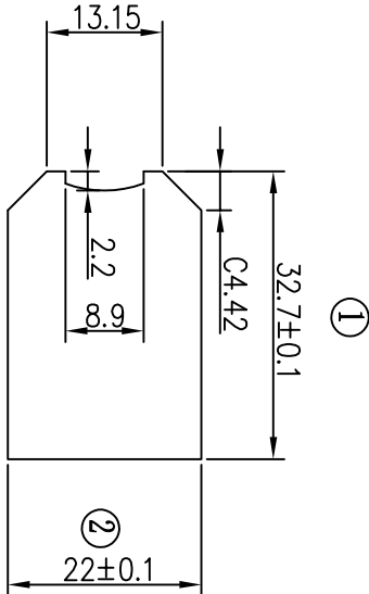
导光板
