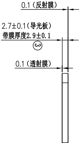
导光板
