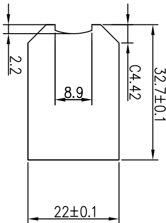
反射膜
